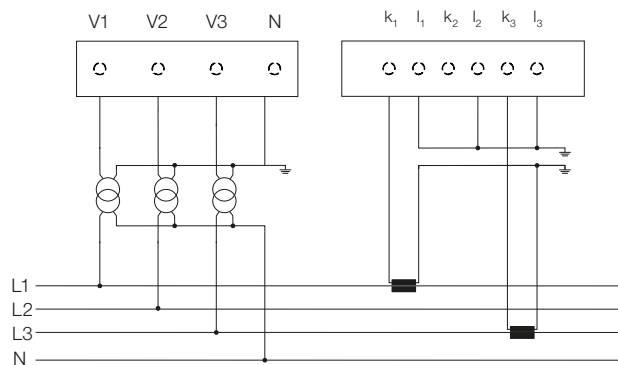
Medición con 3 TP y 2 TCs (ARON) (Válido para MMW03-M22CHB)
