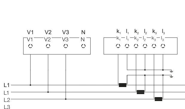
Medición directa de tensión y corriente con 3 TCs
