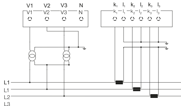
Medición con 2 TP y 3 TCs
