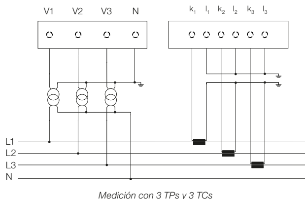
Medición con 3 TP y 3 TCs
