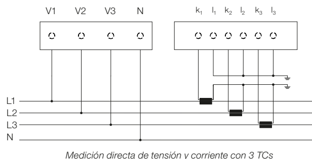
Medición directa de tensión y corriente con 3 TCs
